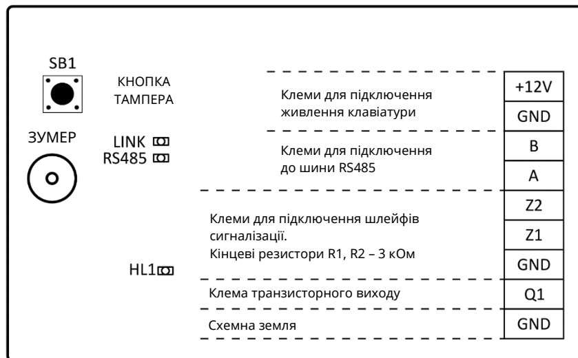
Рисунок А.2 - Схема електрична підключення
