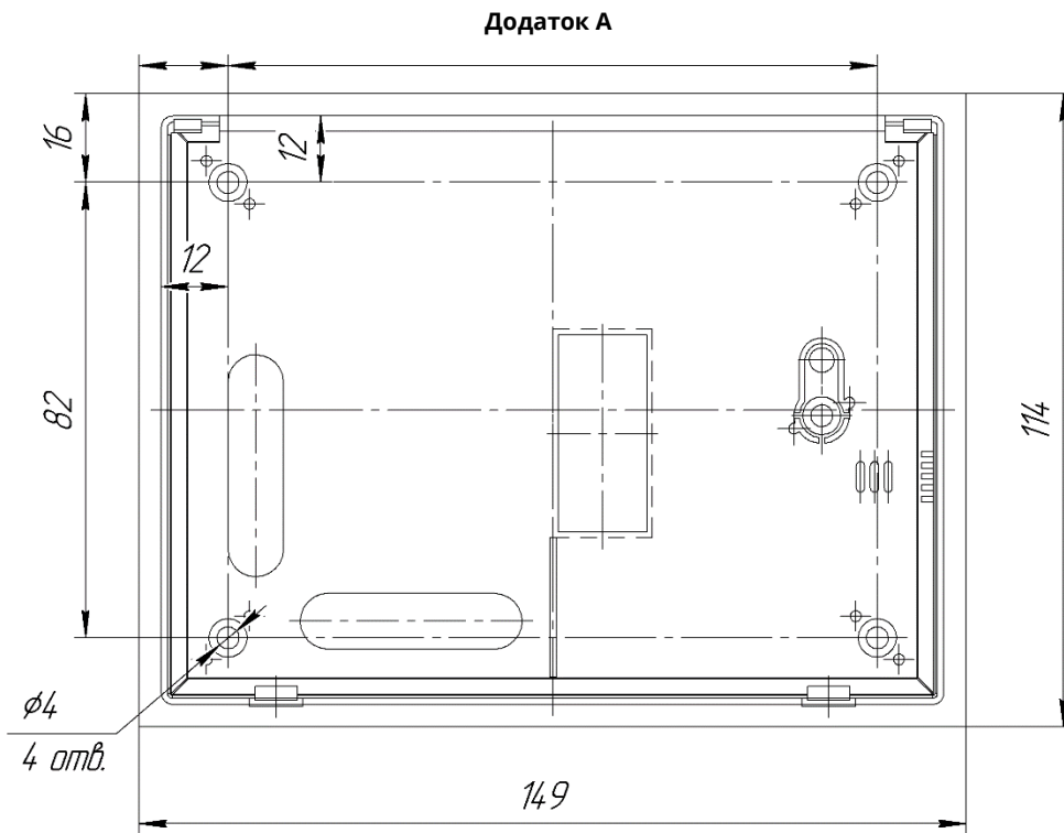
Рисунок А.1 – Установчі розміри клавіатури K-GLCD
