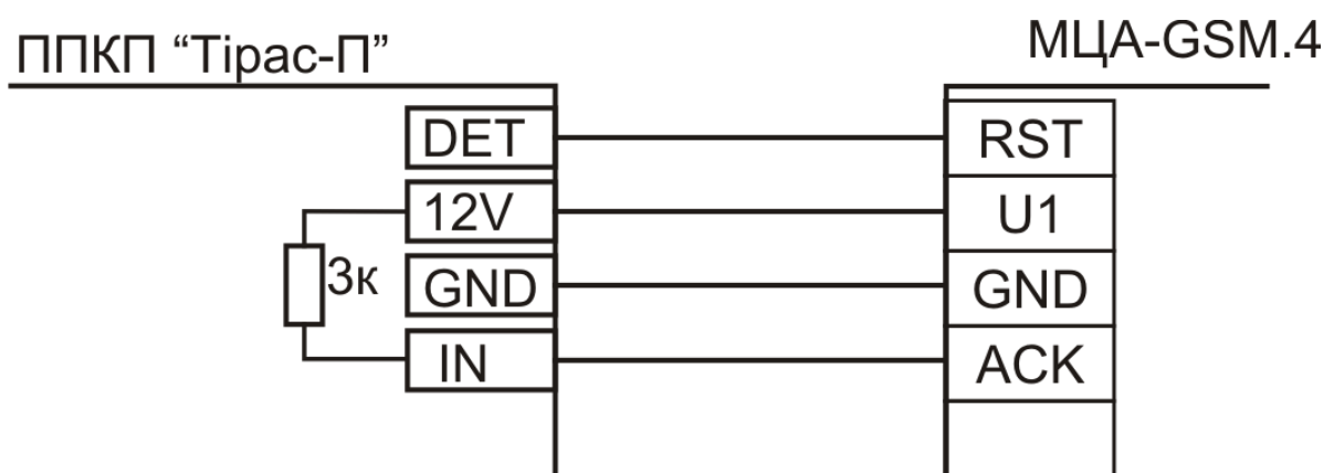
Рисунок В.2 – Приклад підключення входу «RST» та «ACK» (з ППКП «Тірас-4П», Тірас-8П та Тірас-16П).
