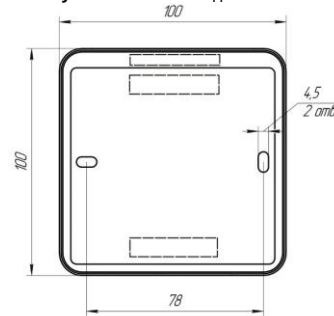
Рисунок А.2 - Розміщення отворів кріплення модуля
