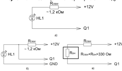
Рисунок А.3 - Схема підключення транзисторного виходу Q1 а - світлодіод засвічується при активації виходу Q1; б - світлодіод працює інверсно до виходу Q1; в - будь-який пристрій зі споживанням до 50 мА.
