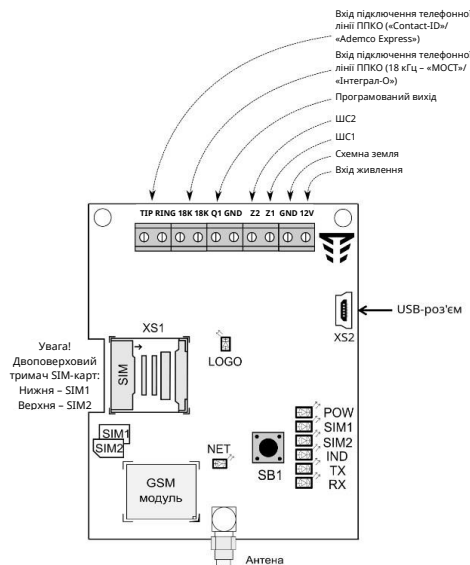
Рисунок А.1 - Схема підключення
