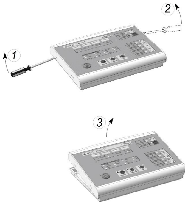
Рисунок 4.2 – Порядок відкривання корпусу ПУіЗ
