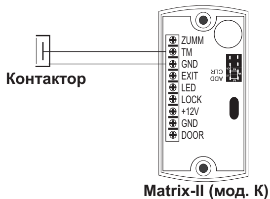
Рис.5 Подключение контактора
