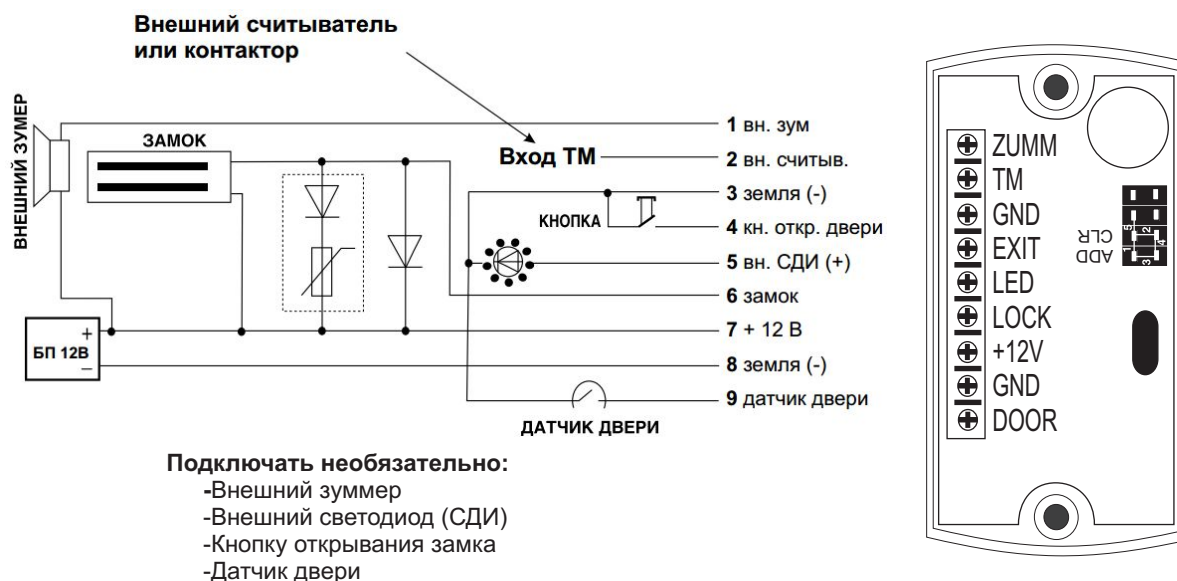
Рис.4 Подключение устройств
