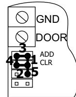
Рис.6 Возможные положения перемычки.
