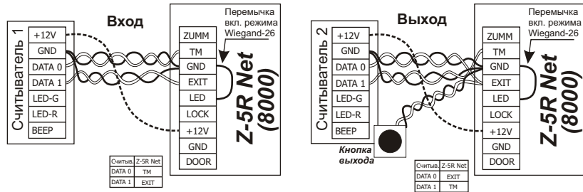
Рис.4 Подключение считывателей к контроллеру по протоколу Wiegand-26
