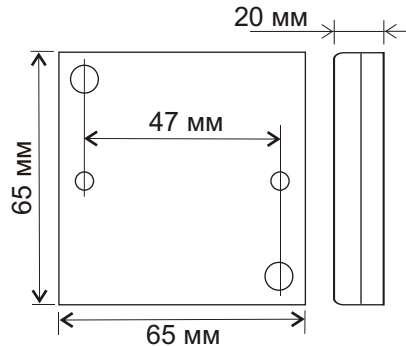
Рис.7 Внешний вид корпуса и габаритные размеры
