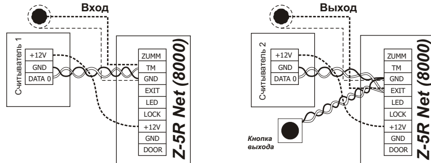
Рис.3 Подключение считывателей к контроллеру по протоколу iButton
