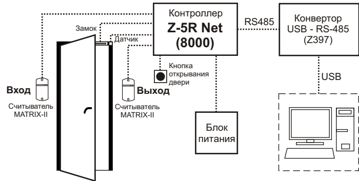
Рис.1 Схема СКУД с контроллером Z-5R Net (8000)
