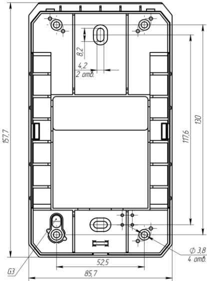
Рисунок 3.1 – Установчі розміри клавіатури Опис елементів плати клавіатури зображено на рисунку 3.2.
